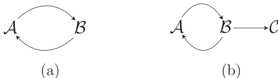
Figura 2.3: Dos AFs y sus extensiones completas.
