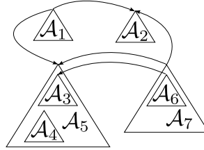
Figura 2.7: Grafo resultante del AF extendido con subargumentos.
