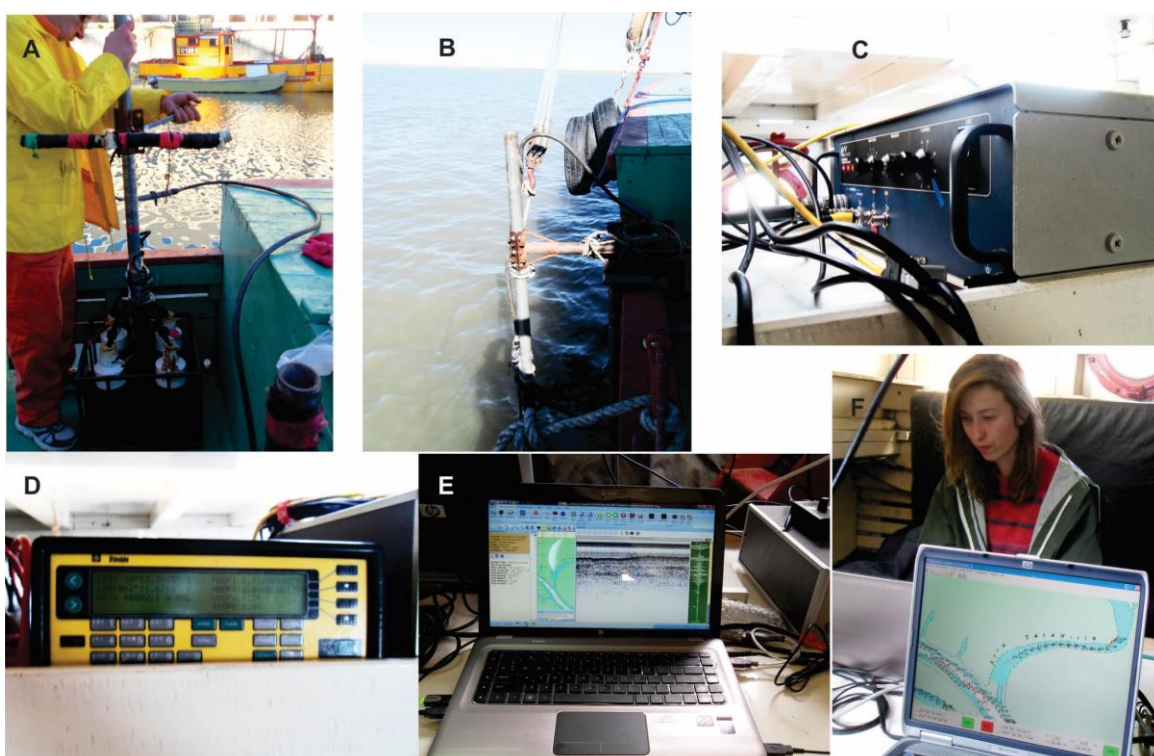
Figura 5. Elementos constituyentes del perfilador sísmico de 3,5 kHz; A) Transductores, B) Estructura soporte de los transductores durante el relevamiento, C) Transmisor del pulso sismo-acústico, D) GPS, E) PC de adquisición y procesamiento de los registros sísmicos en formato digital, F) Navegador empleado para los relevamientos acústicos.
