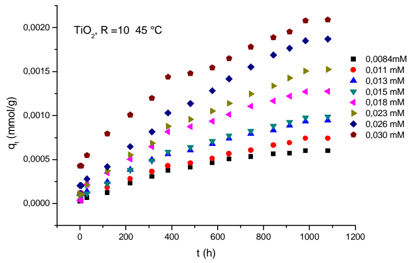
Figura 1: Cantidad adsorbida de MB en función del tiempo sobre R= 10 a 45 °C
