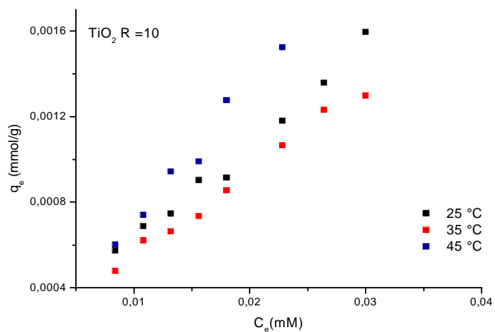
Figura 1: Isotherma de adsorción de MB sobre TiO 2 R= 10
