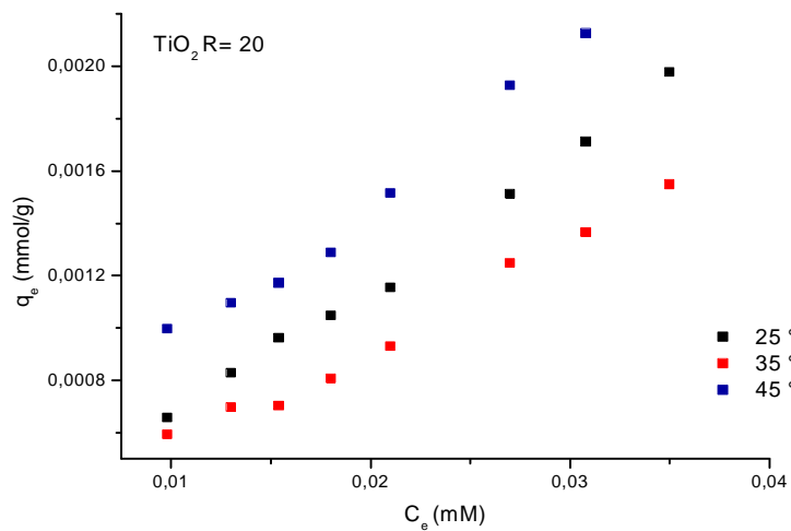
Figura 2: Isotherma de adsorción de MB sobre TiO 2 R= 20
