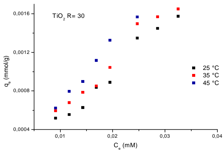
Figura 3: Isotherma de adsorción de MB sobre TiO 2 R= 30
