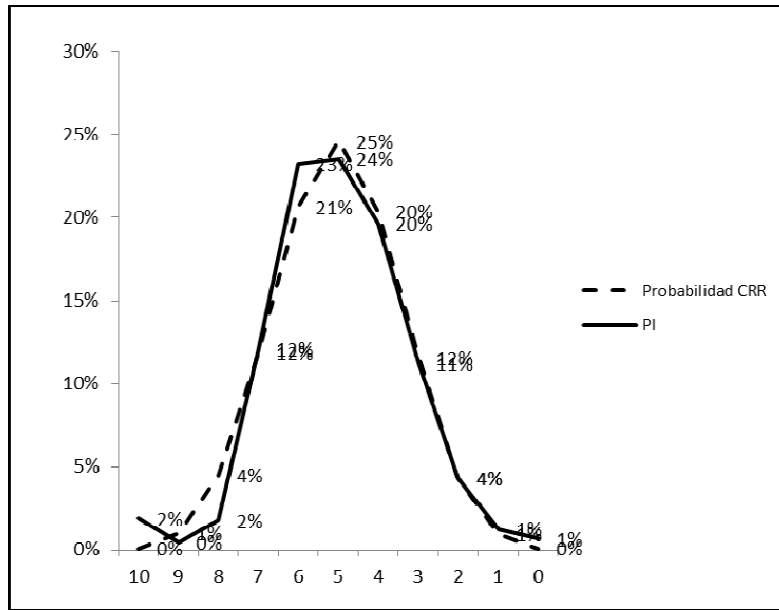
Ilustración 1: Distribución de probabilidades nodos finales
